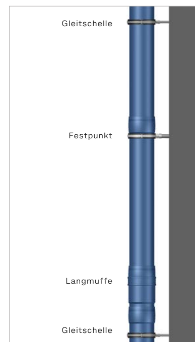
Vertikale Verlegung
